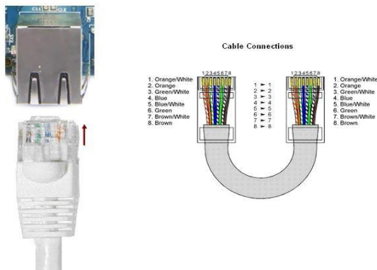
Figure3:Ethernet cable
